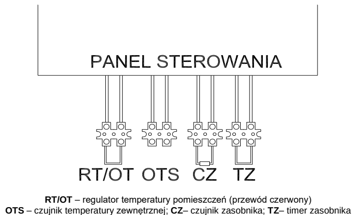
Rys.3.9.1 Płytki sterownika
