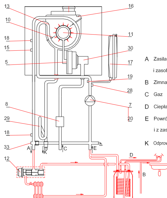
Kocioł jednofunkcyjny
