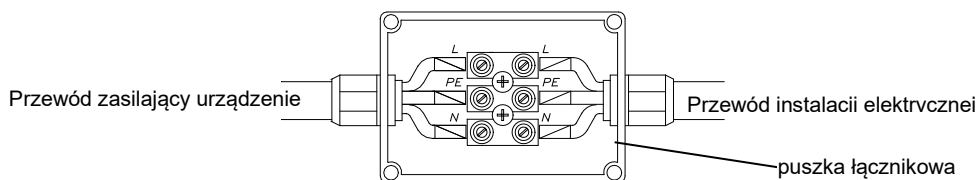
Rys. 3.1.3.1. Kolory żył: L- brązowy; N –niebieski; PE –żółto-zielony
