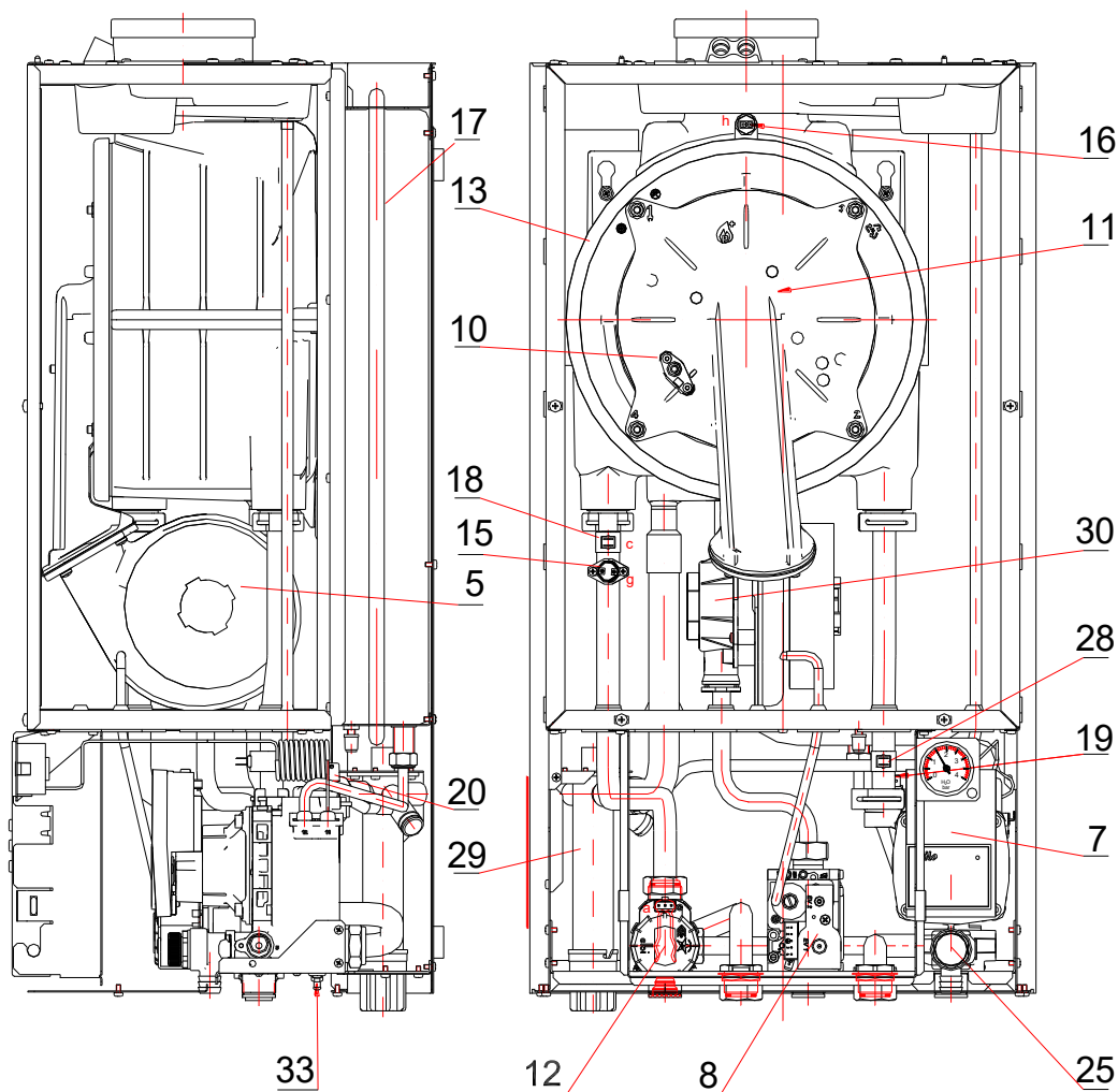
Rys.2.2.1.2. Rozłożenie elementów w kotle ECOCONDENS SILVER jednofunkcyjnym
