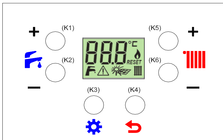
Rys. 5.2.1. Panel sterowania
