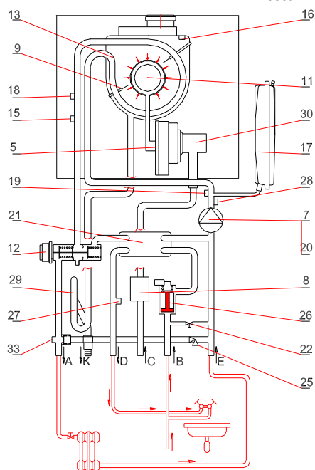
Kocioł dwufunkcyjny
