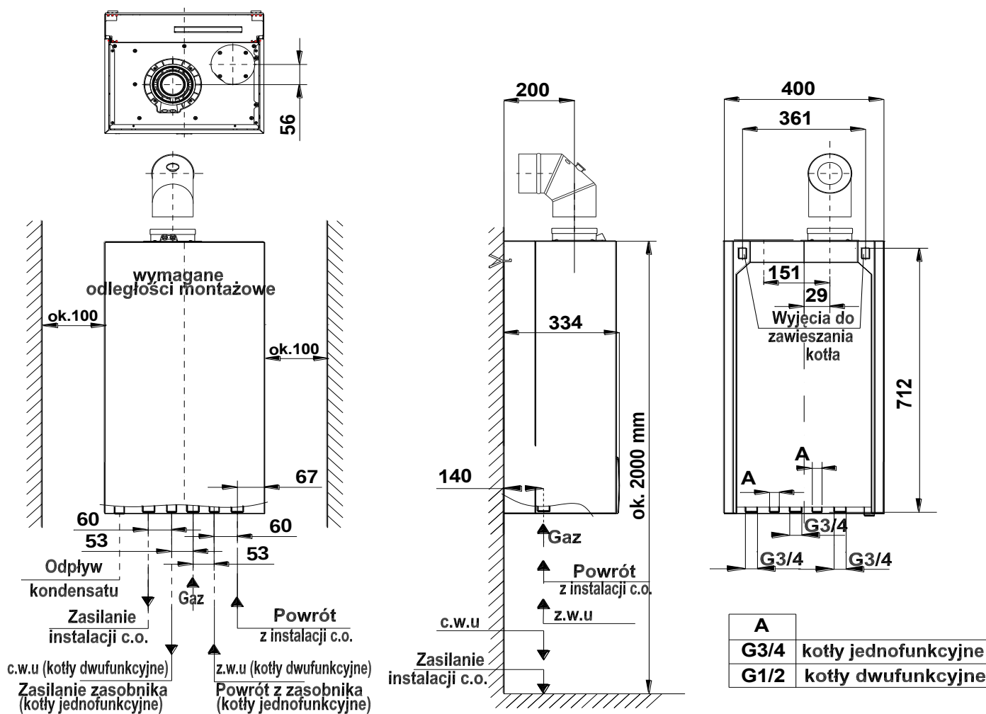
Rys. 3.3.1 Wymiary instalacyjne kotłów ECOCONDENS SILVER
